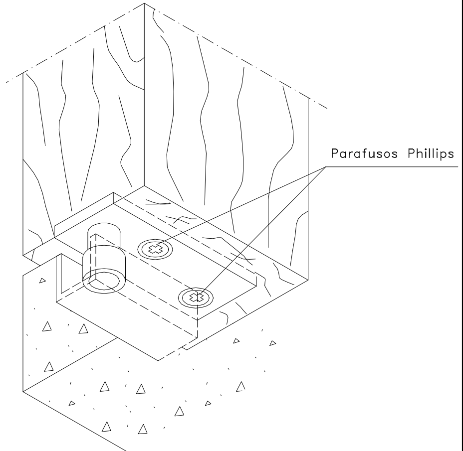
Instalação - escala 1:1
